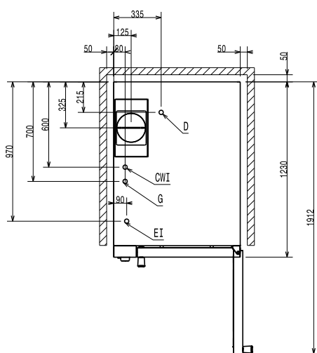
Felülnézet
